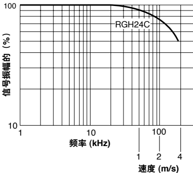
速度 — 模拟类型C读数头 (12 μA)
