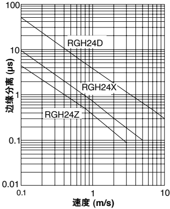
边缘分离 — 数字读数头
