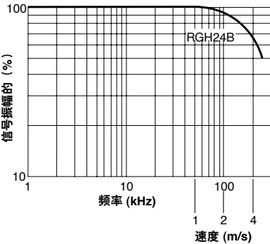
速度 — 模拟类型B读数头 (1 Vpp)
